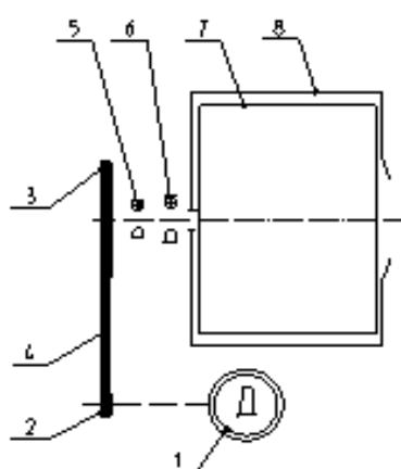
Кинематическая схема машины
