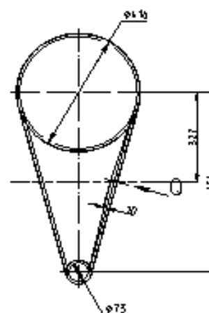
Схема натяжения ремней
