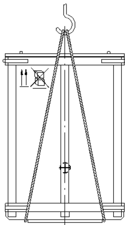
Рис.11. Схема транспортировки
