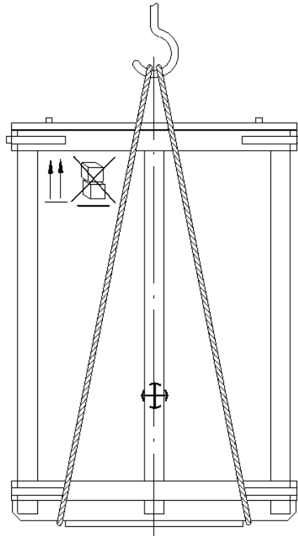
Рис.9. Схема транспортировки
