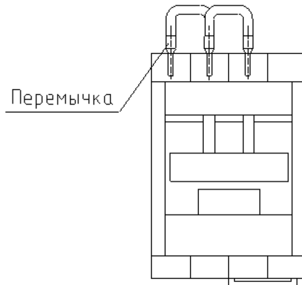
Рис.10 Установка перемычки для подключения ВО-11 к однофазной сети
